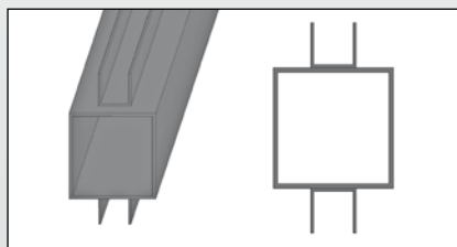
Alu-Pfosten 80 x 80 x 3 mm mit aufgenietetem U-Profil 30 x 30 x 30 x 2 mm pulverbeschichtet, Gerade
