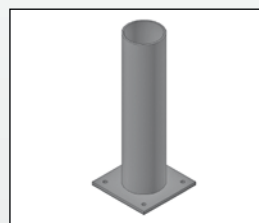
Pfostenbefestigung Ø 73 mm mit Platte 120 x 120 x 8 mm zum Aufdübeln
