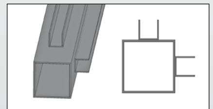
Alu-Pfosten 80 x 80 x 3 mm mit aufgenietetem U-Profil 30 x 30 x 30 x 2 mm pulverbeschichtet, Ecke
